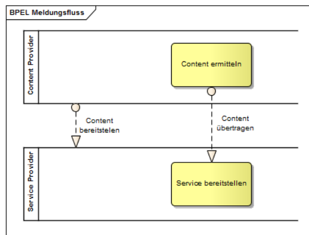
Bild 4-8: BPEL Meldungsfluss
