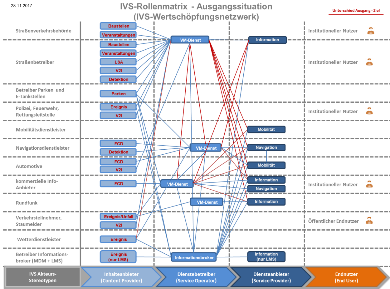
Bild 4-3: IVS-Rollenmatrix – Ausgangssituation
